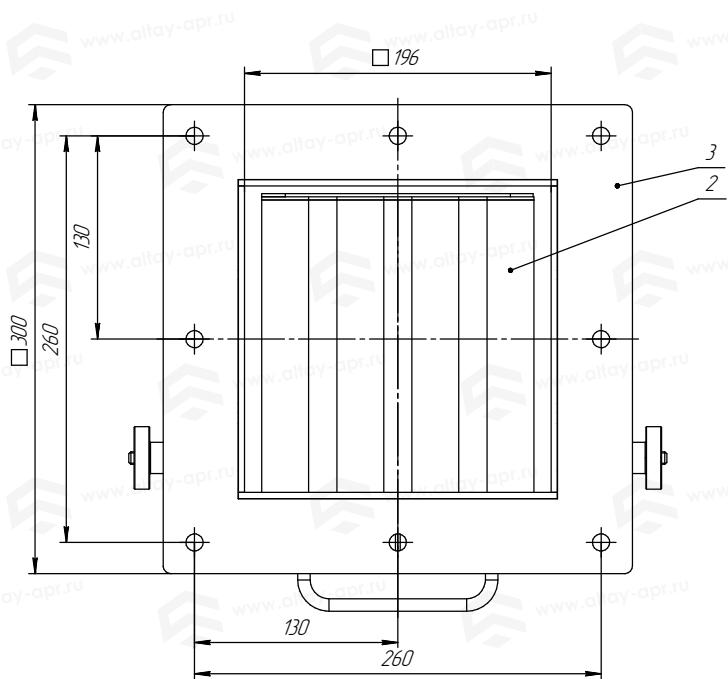
Стержневой сепаратор МС-200
