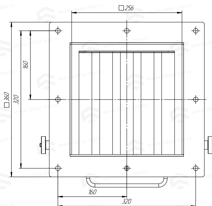
Стержневой сепаратор МС-250
